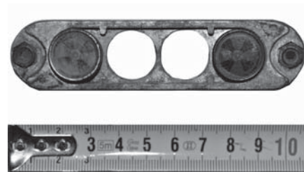
Obr. 5. Signalizátor zavěšení pum z přístrojové desky německé stíhačky Fw 190A. Foto: Z. Schenk
