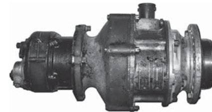
Obr. 3. Setrvačkový startér motoru německé stíhačky Fw 190A. Foto: Z. Schenk
